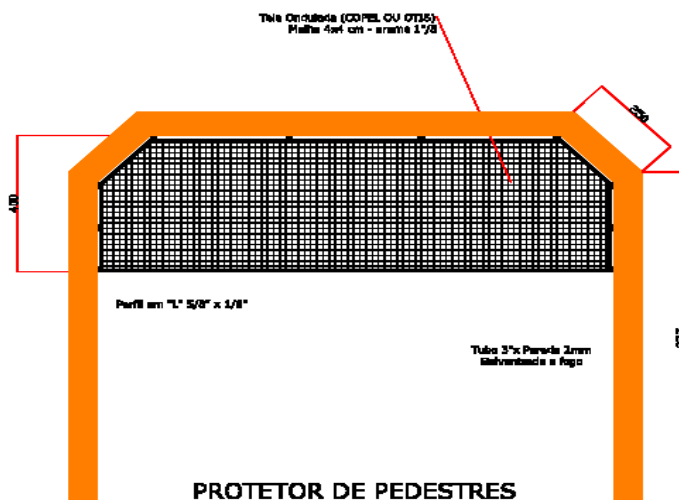
Figura 3: modelo referencial defesa metálica tubular
