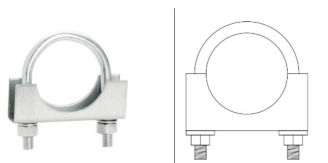
Figura 8: Modelo Referencial Abraçadeira tipo "U"
