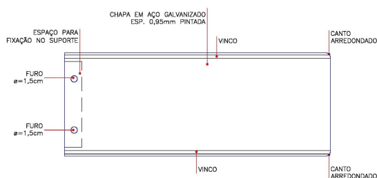
Figura 5: modelo referencial placa toponímia
