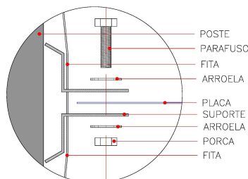
Figura 13: modelo referencial aleta de fixação – detalhe de fixação
