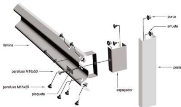
Figura 4: modelo referencial defesa metálica simples
