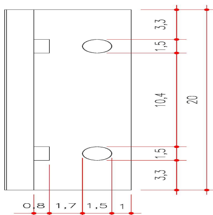
Figura 12: modelo referencial aleta de fixação – vista lateral
