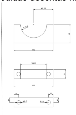
Figura 9: modelo referencial base de apoio
