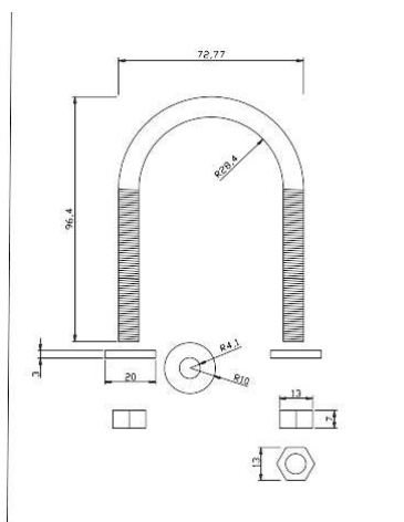
Figura 10: modelo referencial grampo "U"
