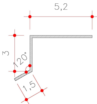
Figura 11: modelo referencial aleta de fixação – vista superior
