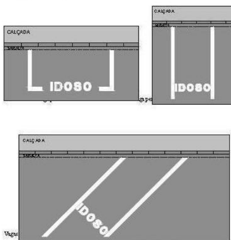
Sinalização horizontal – legenda “IDOSO”
